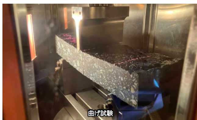
図5 たわみへの追従性評価
