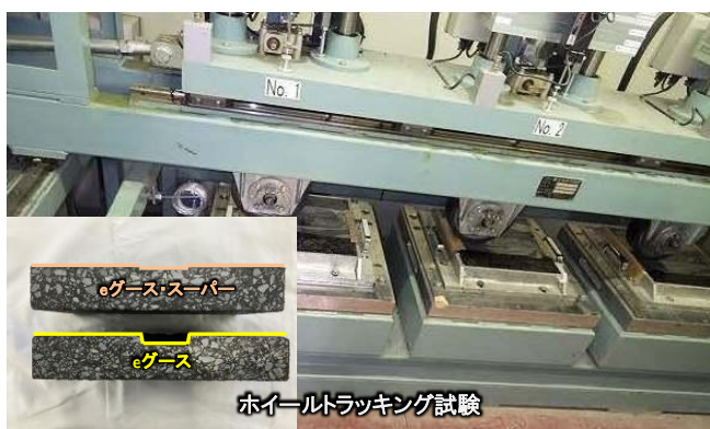
図4 塑性変形抵抗性の評価
